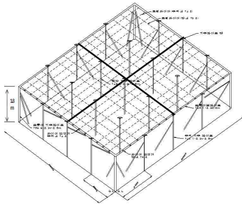
그림 1. 일반형 덕 시설(높이 1.8m)
